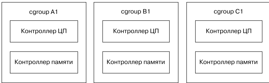
Рис. 8.2. cgroups v2. Процесс может принадлежать только одной группе
